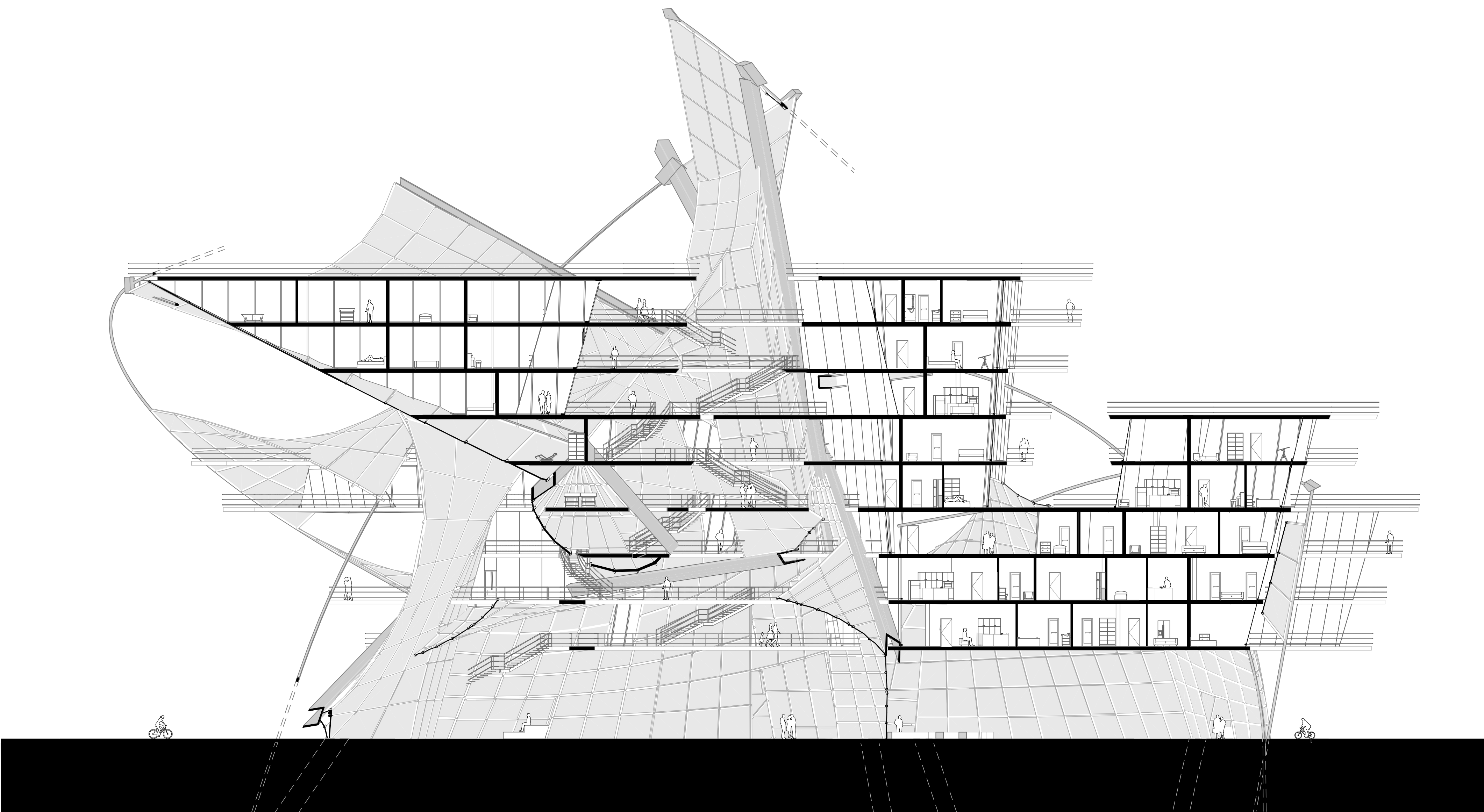
Section A-A
